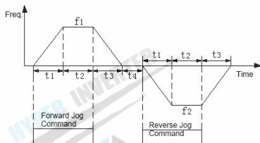
Fig. F1-5 Jog Run
