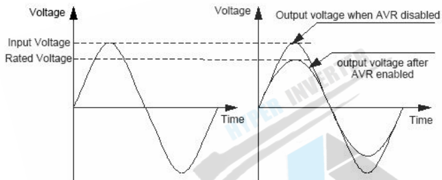
Fig. FC-2 AVR Function
